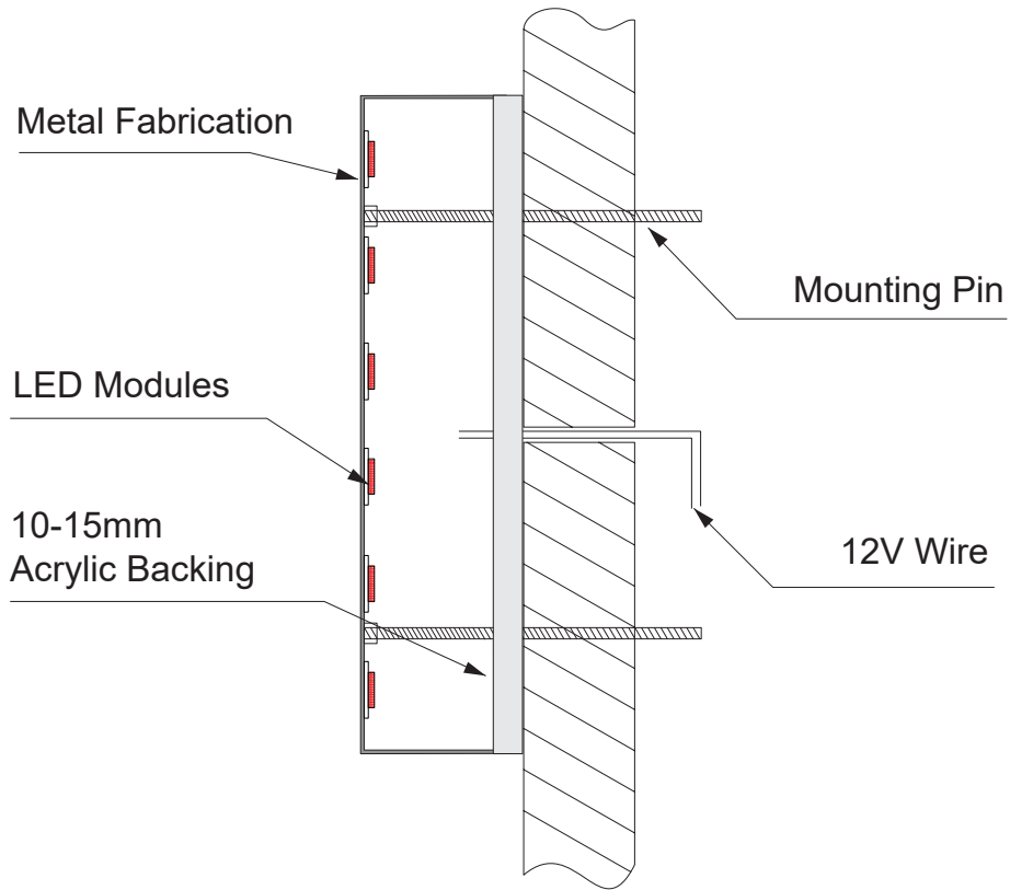
Option A: Flush Mount
