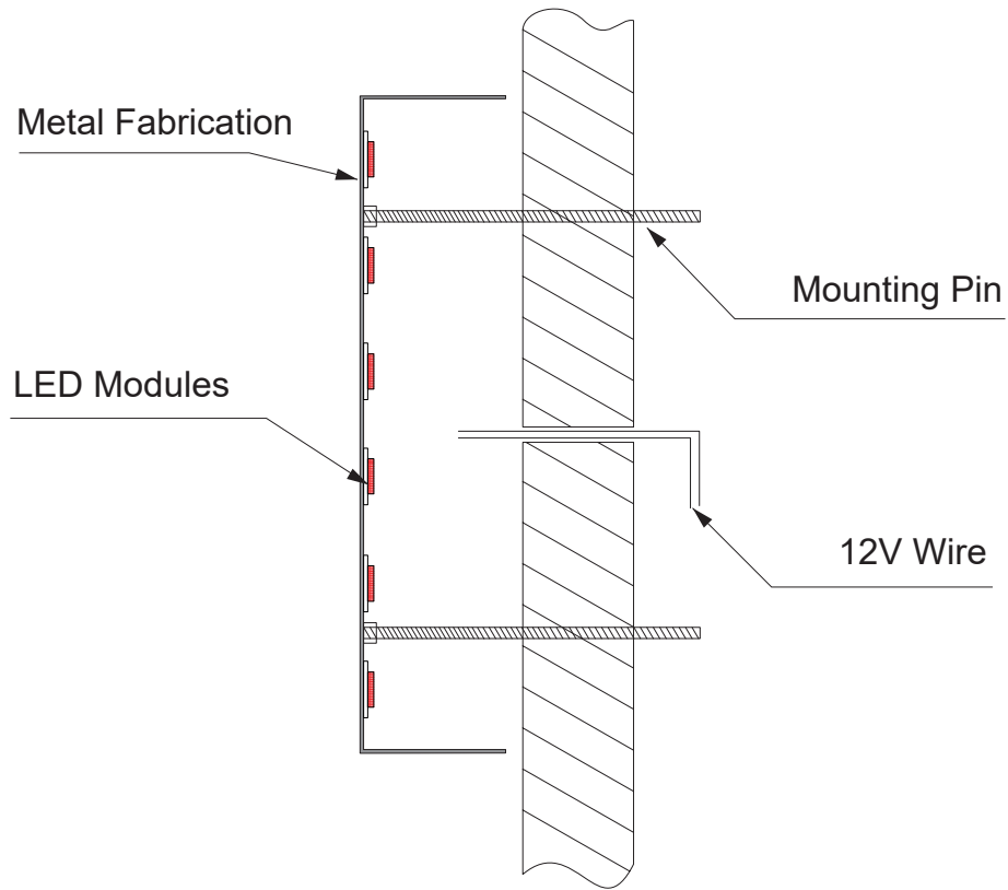
Option A: Open Back
